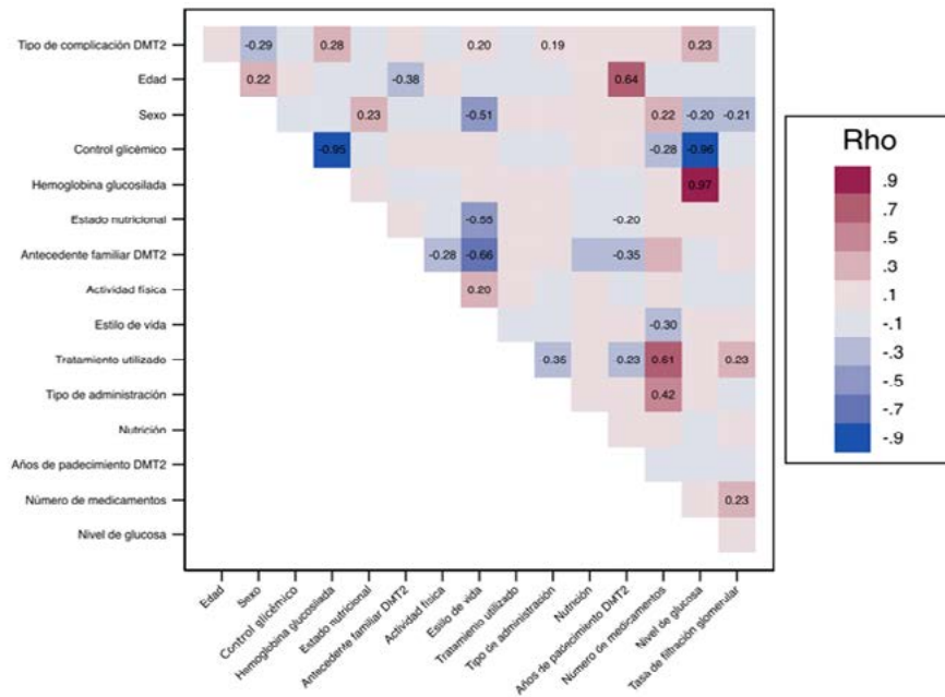
Figura 1. Matriz de correlación policórica / poliserial de factores de estudio. Se muestran las correlaciones estadísticamente significativas ( p < 0.05 ).
