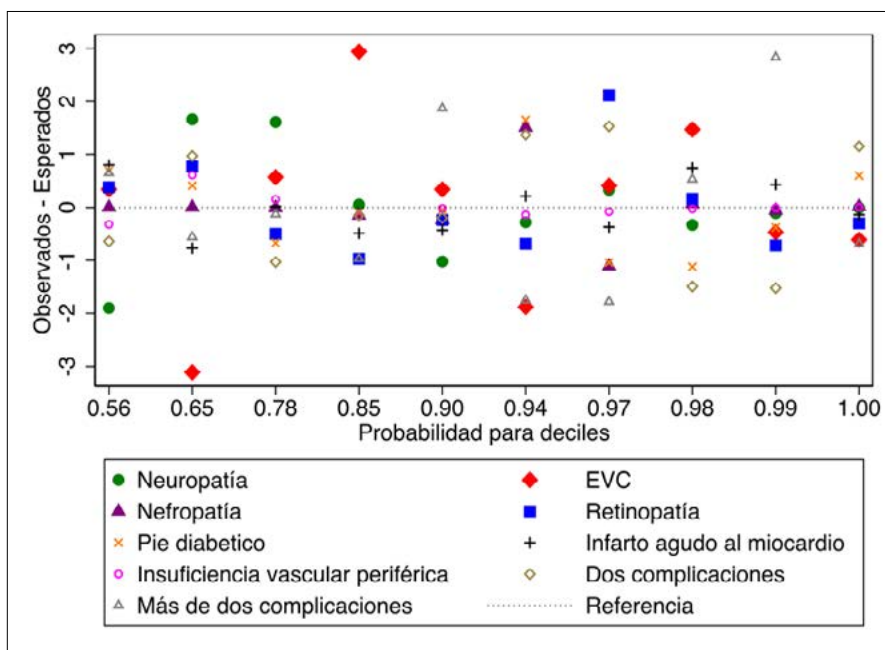
Figura III. Diferencia de observados y esperados con MRLM-Bootstrap final.
