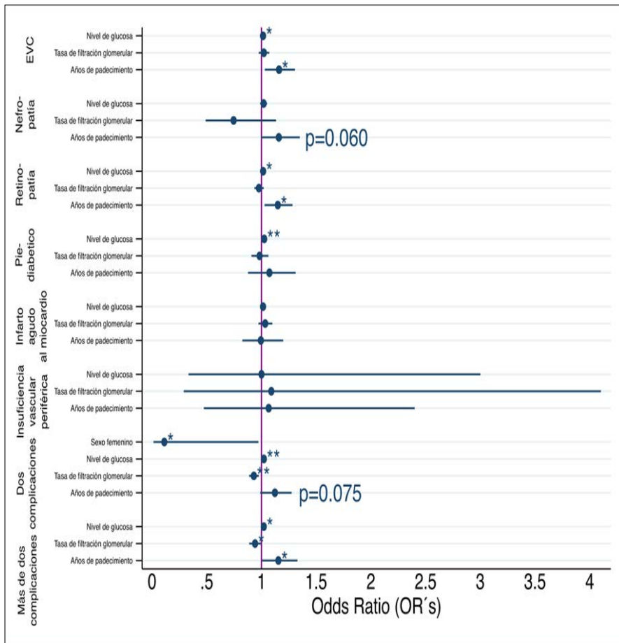
Figura II. Factores de riesgo para complicaciones de DMT2 usando el MRLM-Bootstrap final.
